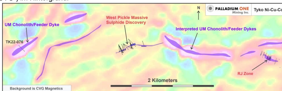
Abbildung 3. Lageplan der Zonen West Pickle und RJ mit Maxwell-Platten der elektromagnetischen (EM) Flug- und Bodenmessungen mit errechnetem vertikalem Gradienten der Magnetfeldstärke (Calculated Vertical Gradient Magnetics, „CVG“) im Hintergrund.
