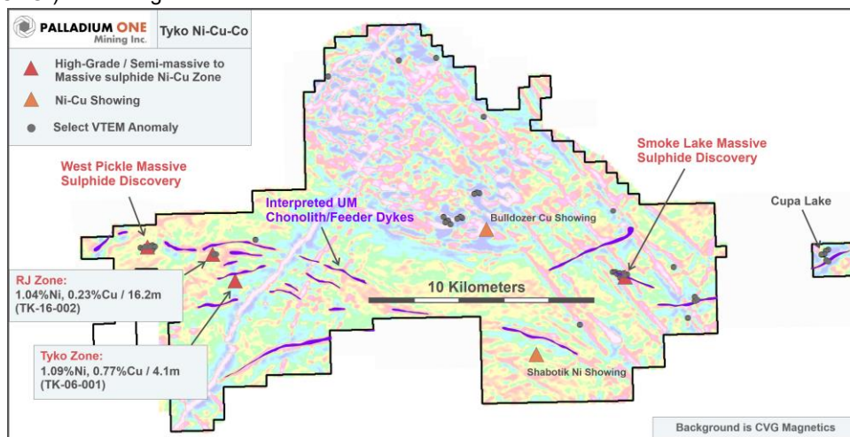
Abbildung 2. Lageplan des Konzessionsgebiets Tyko mit verschiedenen mineralisierten Zonen und VTEM-Multi-Line-Anomalien mit errechnetem vertikalem Gradienten der Magnetfeldstärke (Calculated Vertical Gradient Magnetics, „CVG“) im Hintergrund.
