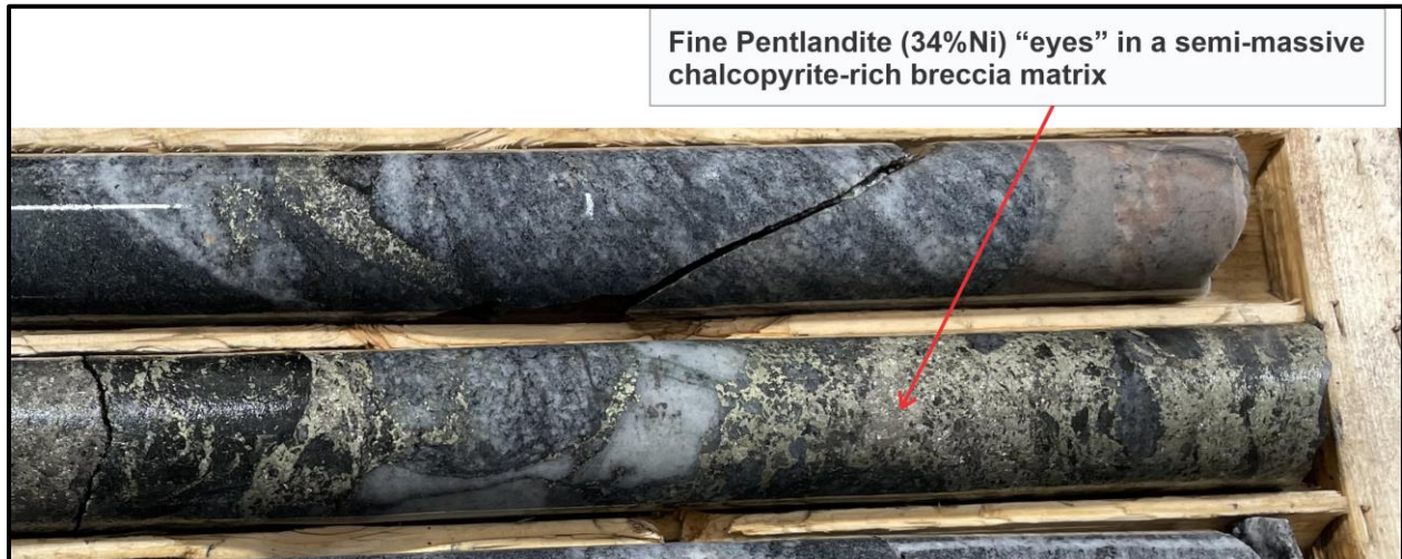
Abbildung 2. Semi-massive Pentlandit-Pyrrhotin-Chalkopyrit-Sulfid-Mineralisierung in Bohrloch TK-22-059.
