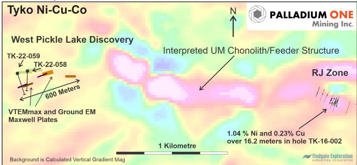
Figure 4. Vergrößertes Plandiagramm der Zone RJ und der neuen Zone West Pickle mit Maxwell-Plates der VTEMmax- und Bodenuntersuchungen an der EM mit errechneter vertikaler Steigung (Calculated Vertical Gradient, „CVG“) im Hintergrund.
