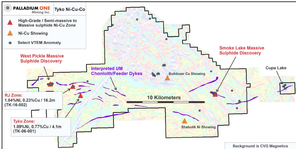
Abbildung 3. Karte der Liegenschaft Tyko mit Darstellung mehrerer (einschließlich West Pickle) hochgradiger und massiver Sulfid-Nickel-Kupfer-Zonen (Dreiecke) in und neben einem Camp interpretierter ultramafischer Feeder-Gänge (violett).
