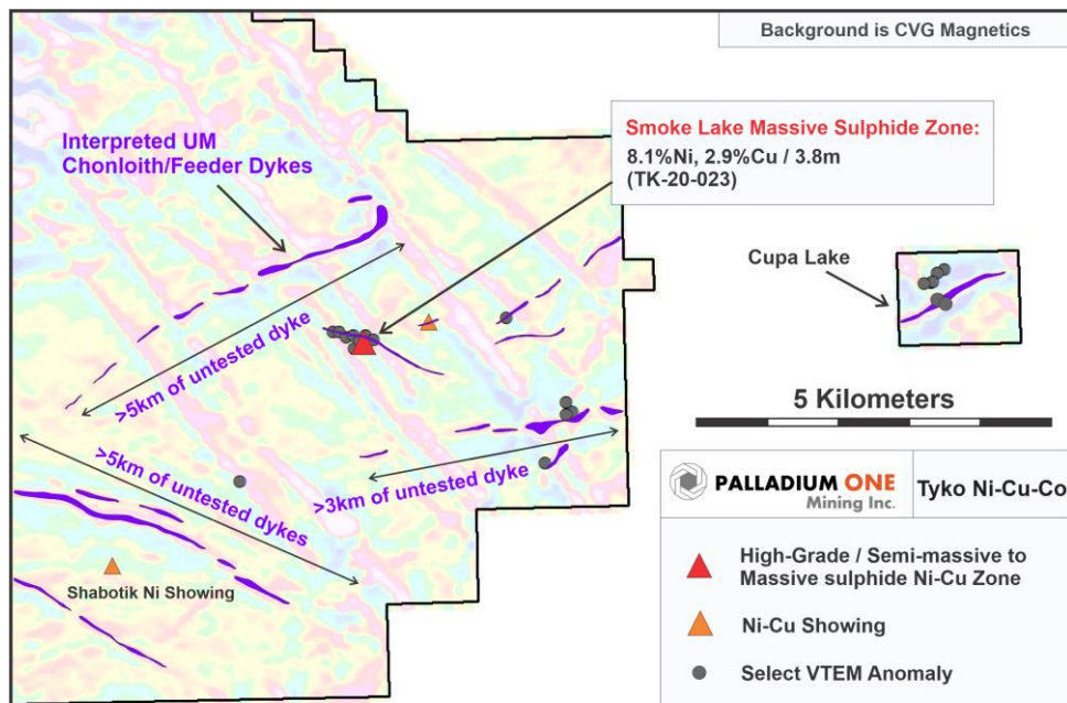
Abbildung 5. Karte der Liegenschaft Tyko ( Ostseite der Liegenschaft ) mit Darstellung der hochgradigen massiven Sulfid-Nickel-Kupfer-Zone Smoke Lake in und neben einem Camp interpretierter ultramafischer Feeder-Gänge (violett).
