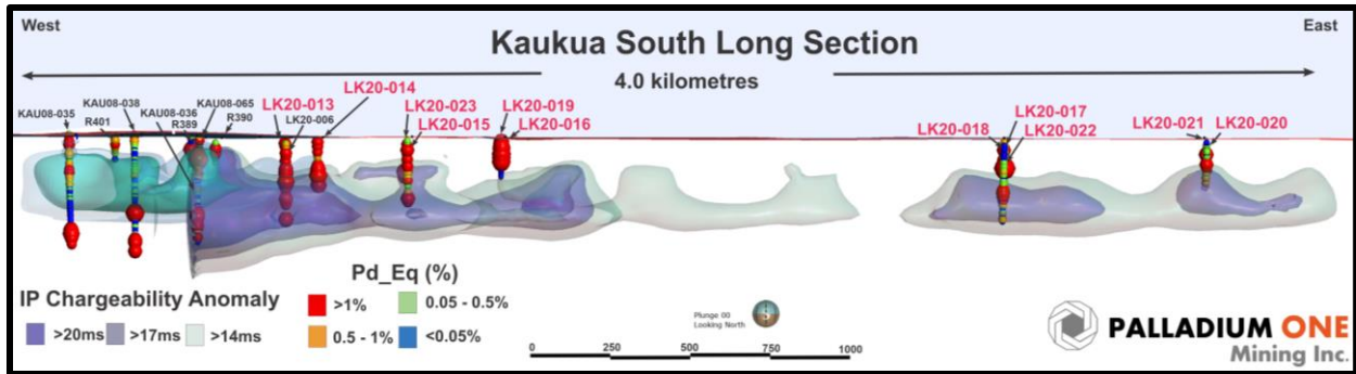
Abbildung 3 Querschnitt durch Kaukua South, mit Blick Richtung Westen auf die Bohrlöcher LK20-016 und -019.
